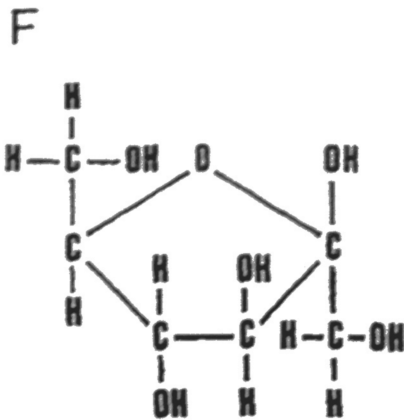
Fructose
