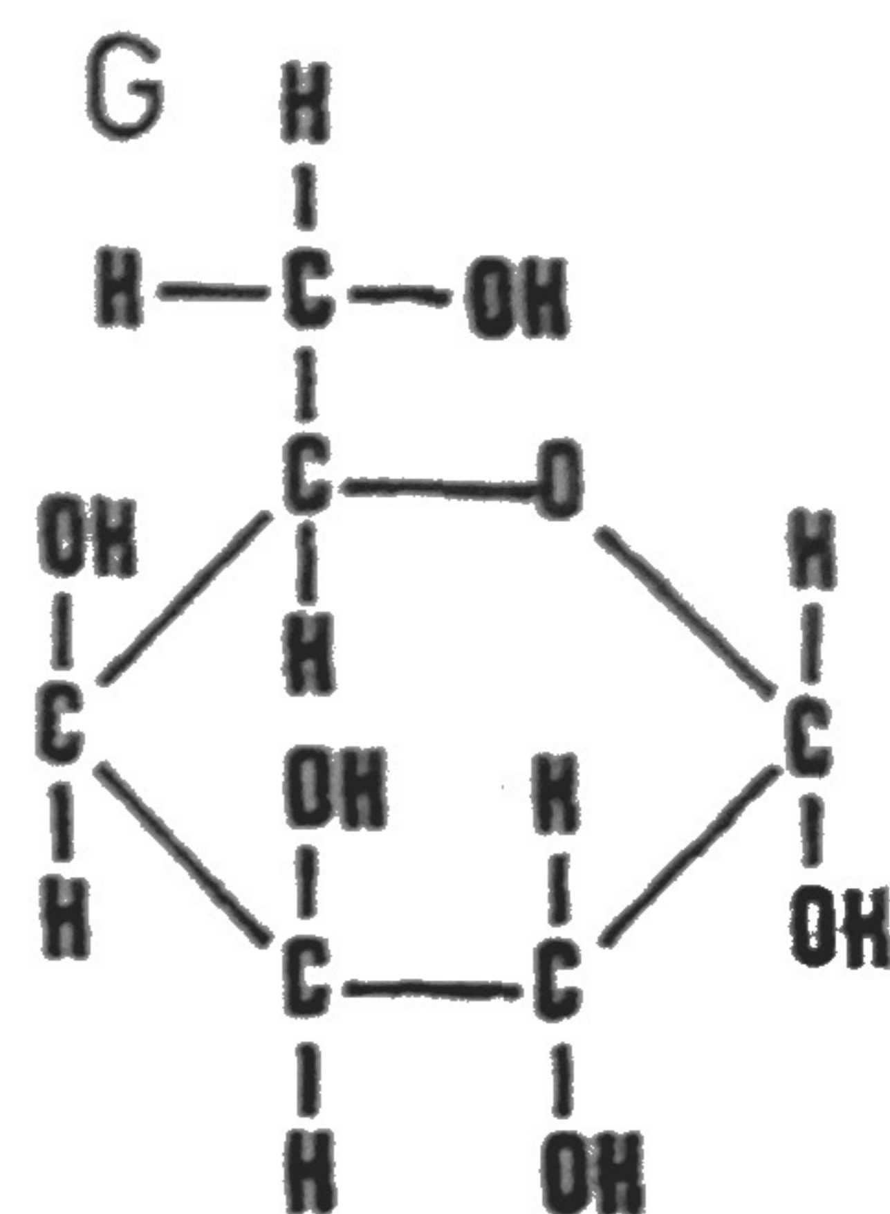
Galactose
